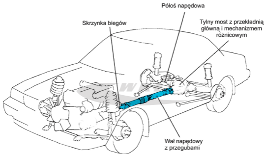
Rys. 1.15 Klasyczny układ przeniesienia napędu [59]
