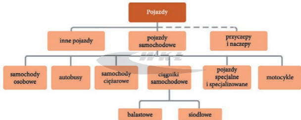
Rys. 1.1 Klasyfikacja pojazdów
