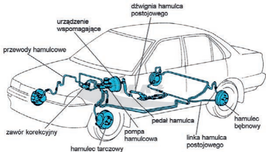
Rys. 1.16 Układ hamulcowy samochodu osobowego [58]
