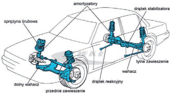
Rys. 1.14 Zawieszenie samochodu osobowego [58]
