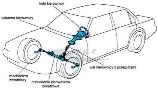
Rys. 1.15 Układ kierowniczy samochodu osobowego [58]
