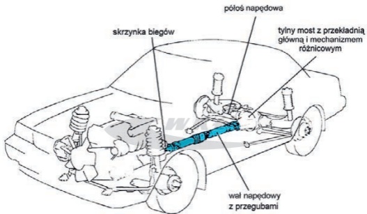
Rys. 1.13 Klasyczny układ przeniesienia napędu [65]
